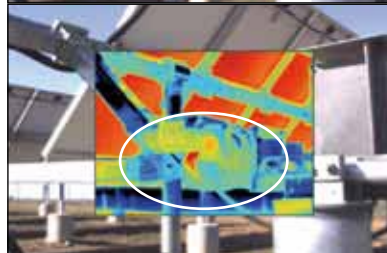
Verificación térmica de los motores del seguidor
