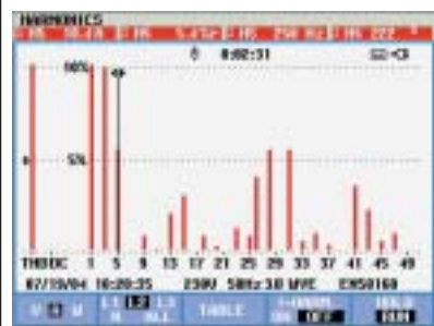
Figura 5 - Tensión y corriente en una batería de condensadores. Espectro de corriente
