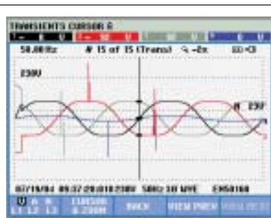
Figura 1 - Transitorios en una red.
